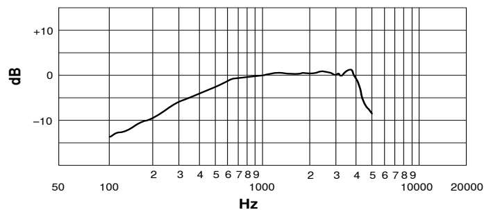
RISPOSTA IN FREQUENZA TIPICA
