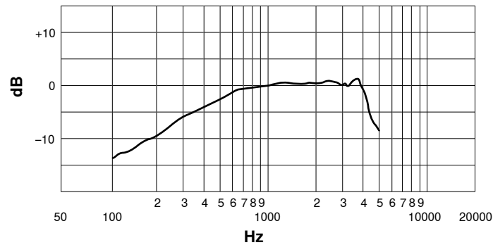
TYPISCHER FREQUENZGANG
