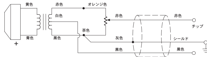
内部接続
