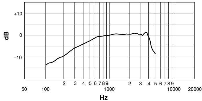
RESPUESTA DE FRECUENCIAS TIPICA
